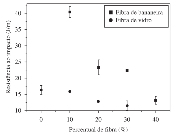
Figura 4. Resistência ao impacto do HDPE com fibras de bananeira e de vidro em diferentes percentuais em massa.
