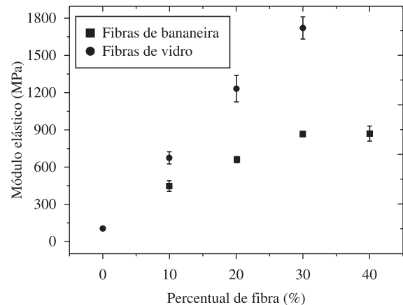
Figura 2. Módulo elástico do HDPE com fibras de bananeira e de vidro em diferentes percentuais em massa.
